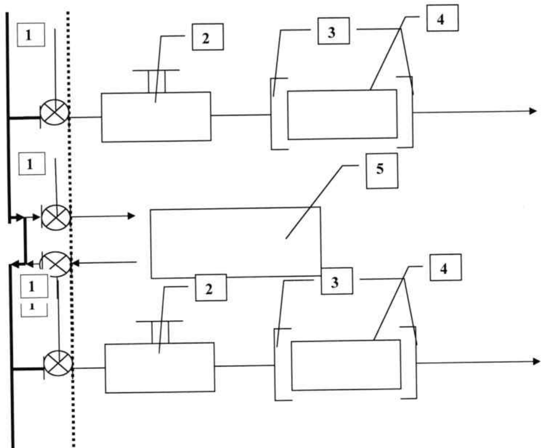
Схема ГВС
